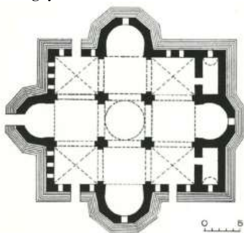
Figure 25. Plan d'une église arménienne
