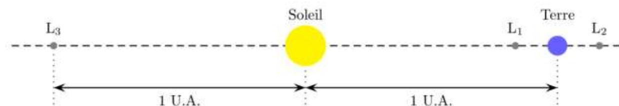
Schéma 1. Position du point de Lagrange par rapport aux positions du soleil et de la terre
