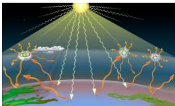
Figure 3. Principe de l'effet de serre
