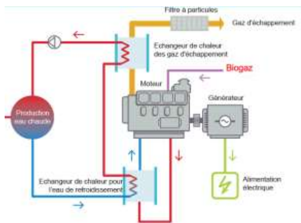
Figure 7. Principe de la cogénération
