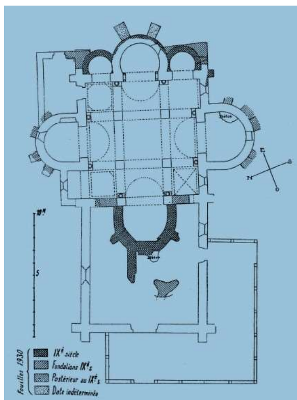
Figure 24. Plan de l'oratoire carolingien de Germigny des Prés
