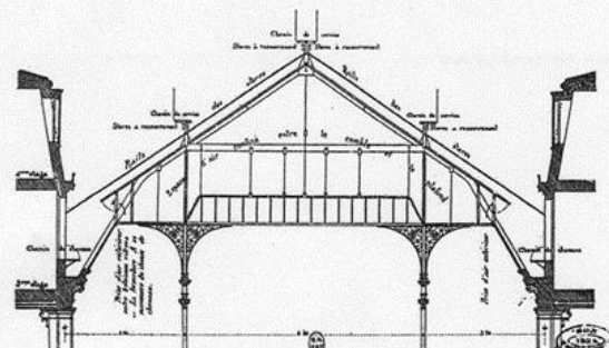
N° 106 Coupe d'une lanterne.
