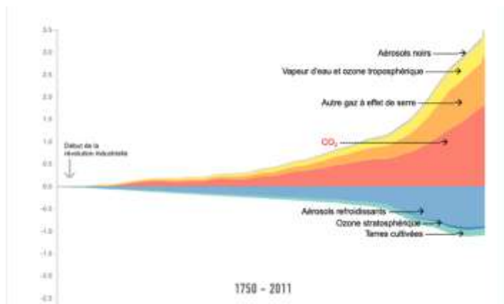
Figure 5. Contribution de l'activité humaine à l'effet de serre
