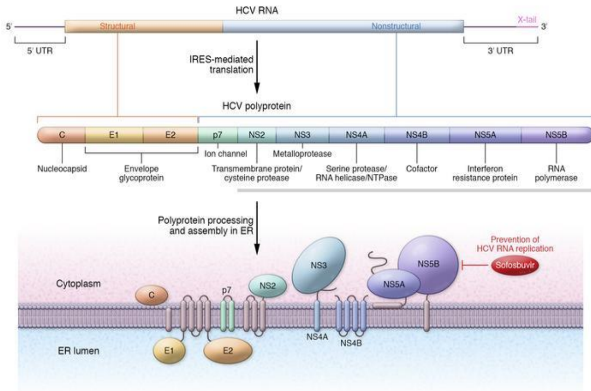
Figure 4. Schéma du génome viral (ARN+) du virus de l'hépatite C et schéma de la polyprotéine qui, après coupure par des protéases s'organise sous forme d'une dizaine de protéines autour de la membrane du réticulum endoplasmique à l'intérieur de la cellule R. Bartenschlager, C. Rice, M. Sofia J Clin Invest. 2016;126(10):3639-3644. https://doi.org/10.1172/JCI90179
