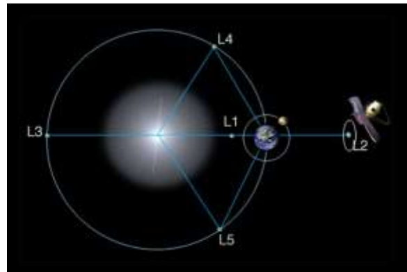
Figure 2. Le point L2, l'un des cinq points de Lagrange
