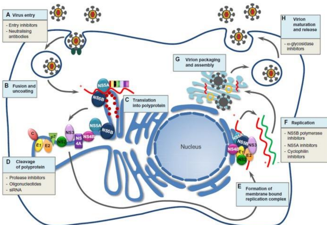
Figure 5. Schéma récapitulatif de l'entrée, de la formation et de la sortie du virus dans une cellule animale. P. de Leuw, C. Stephan, GMS Infect Dis. 2017 ; doi: 10.3205/id000034
