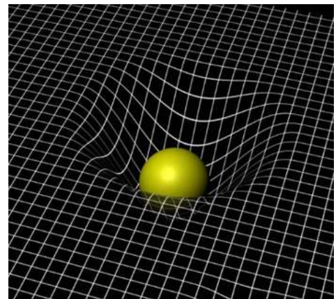
Détection des ondes gravitationnelles
