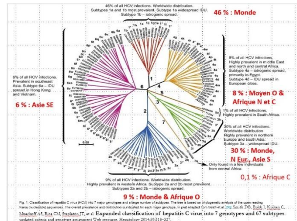
Figure 3. Classification des 7 génotypes et 67 sous-types du virus de l'hépatite C en 2014
