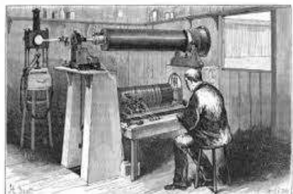
Fig. 4 La machine de Cornu. A gauche la source de lumière et sur le portant le système électro- mécanique de rotation de la roue dentée. A droite en haut le cylindre qui contient l'optique collimatrice qui envoie et reçoit le faisceau lumineux et en dessous le système d'enregistrement graphique.
