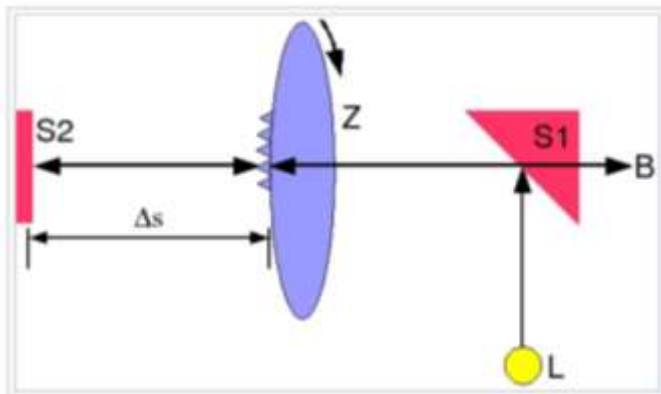
Fig. 2 – Mesure de la vitesse de la lumière. Expérience de Fizeau. La lumière collimatée émise par la source L est réfléchi par le prisme S1 et passe entre deux fines dents de la roue Z qui génère ainsi des éclairs qui se propagent jusqu'au miroir S2 distant de \Delta s . Les éclairs sont renvoyés par le miroir S2 vers la roue dentée. Selon la vitesse de la roue et le nombre de dents, les éclairs lumineux en retour sont bloqués par une dent ou passent par le creux suivant. Le temps mis par une dent pour s'interposer est aussi le temps mis par la lumière pour un aller-retour. Le temps étant connu ainsi que la distance, on en déduit la vitesse de la lumière.
