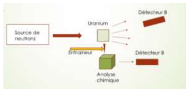
Fig.8 Principe de détection des espèces produites lors du bombardement d'une cible d'uranium par des neutrons
