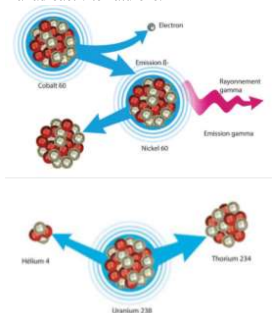
Fig. 1 - La radioactivité naturelle. Exemples du Cobalt 60 et de l'Uranium 238
