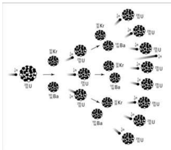
Fig.11 Réaction de fission en chaîne
