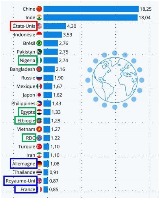
Figure 3. Populations relatives de divers pays (en %), d'après l'ONU.
