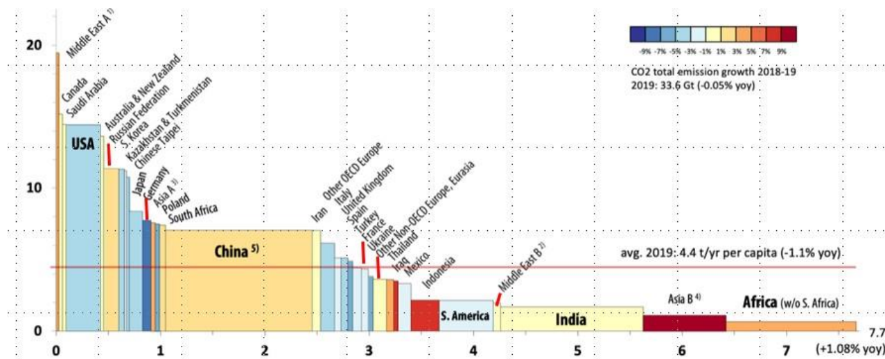
Figure 2. Vue générale de l'émission de CO 2 dans différents pays. En ordonnée, l'émission de CO 2 en tonnes par habitants, en abscisse le nombre d'habitants dans le pays.
