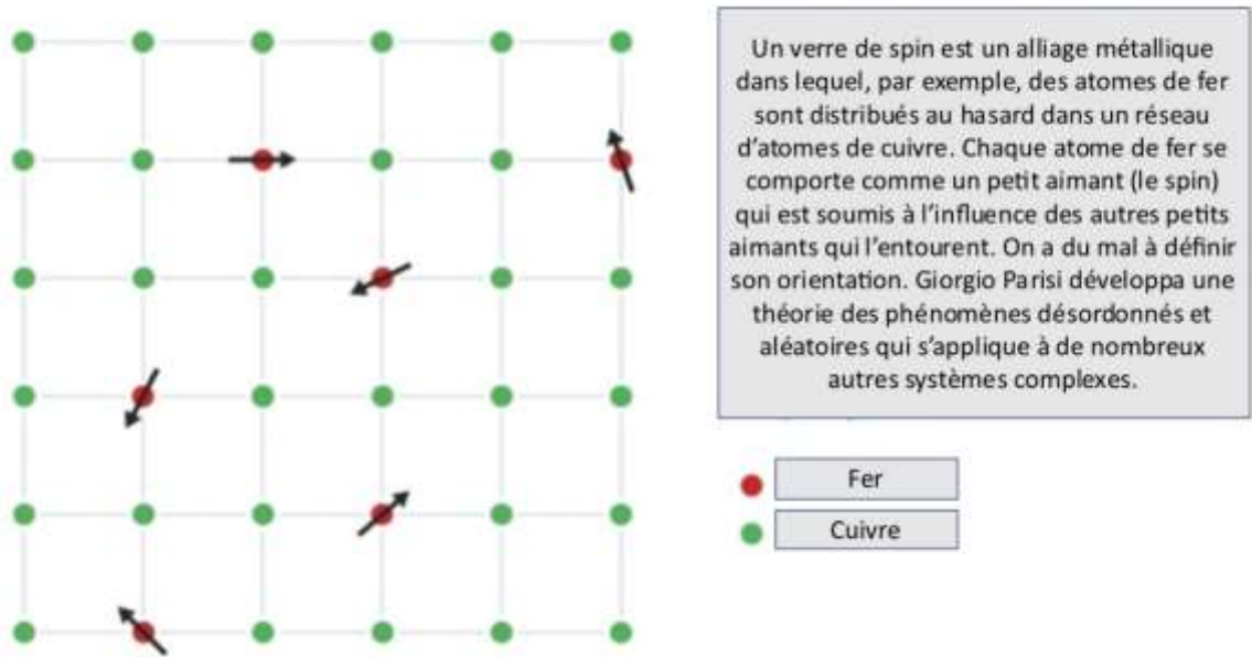
Figure 4. Structure atomique d'un verre de spin
