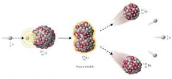
Fig. 10 Modèle de la goutte d'eau de l'atome d'uranium. Le neutron n entre en collision avec le noyau d'uranium U 235 qui se déforme, devient instable puis se scinde en deux noyaux plus légers, le baryum Ba 141 et le krypton Kr 92 avec l'émission de 3 neutrons de grande énergie.
