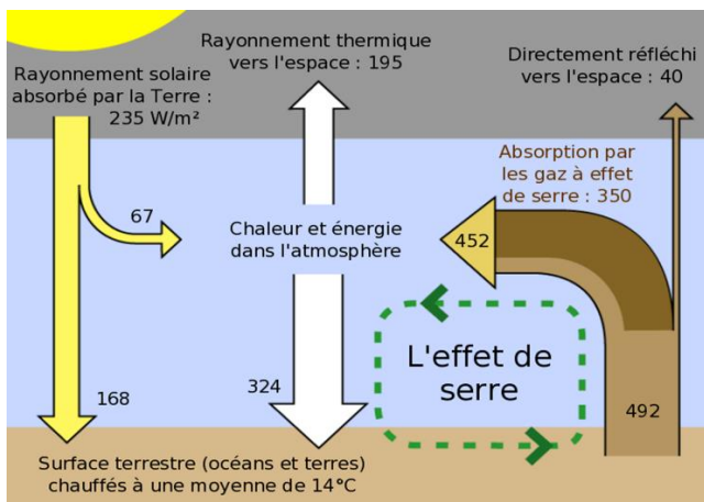
Figure 1. Les échanges thermiques incluant l'effet de serre. https://www.techno-science.net/
