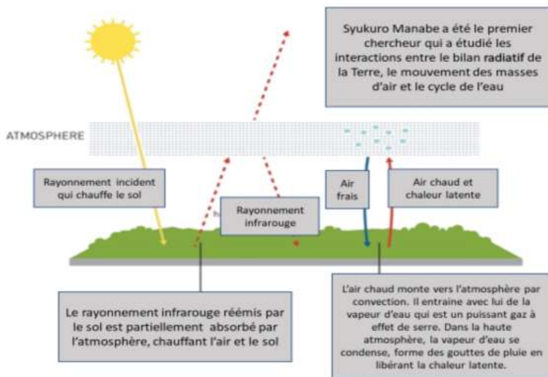
Figure 2. Modèle de climat de Manabe
