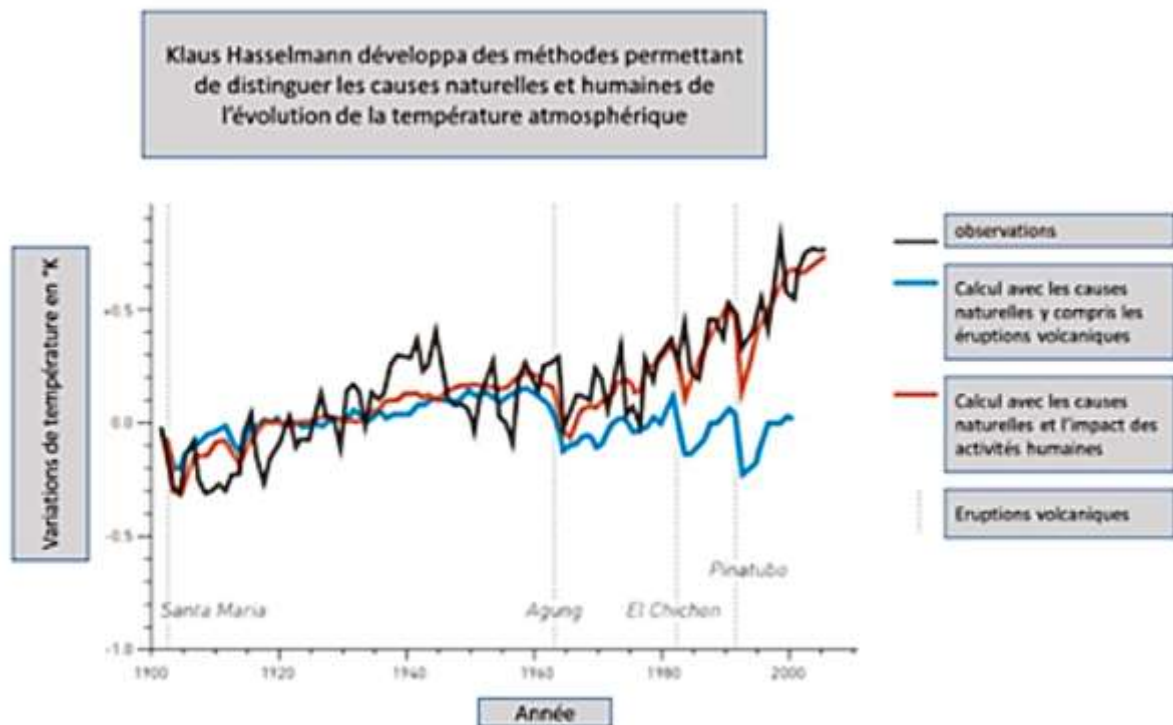
Figure 3. Variation de la température atmosphérique. Calculs calés sur la moyenne des températures observées entre 1901 et 1950
