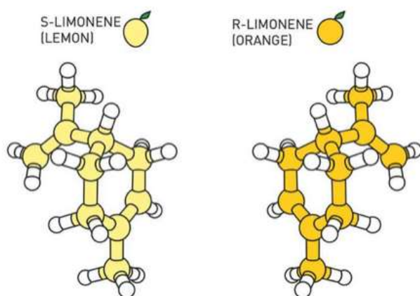
Figure 6. Les deux formes du limonène et
