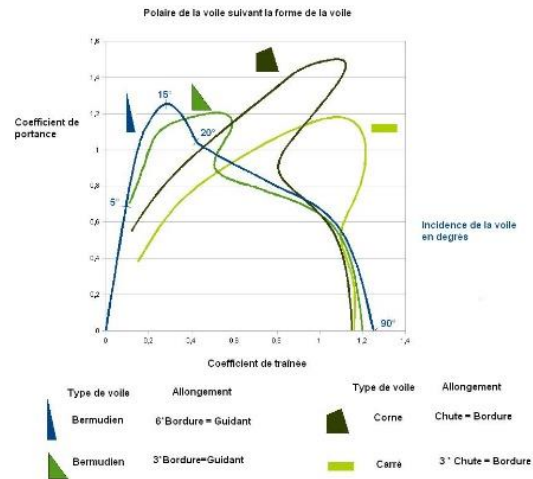
Figure 17. Polaires de voiles typiques
