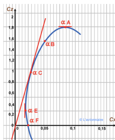
Figure 15. Polaire aérodynamique d'un profil
