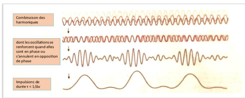
Pour fabriquer une impulsion \tau , il faut combiner des harmoniques dont la période d'oscillation est \leq \tau et la fréquence \geq 1/\tau . Donc des harmoniques de rang élevé dans une bande de fréquence \Delta\nu > 1/\tau
