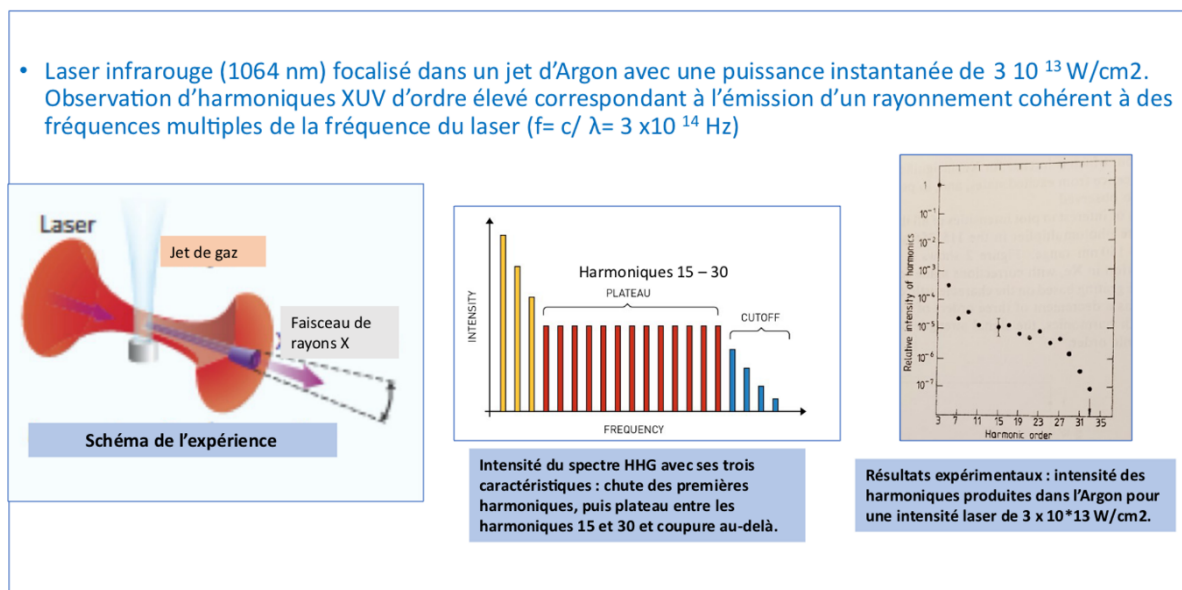
Figure 6 - Génération d'harmoniques de rang élevé (HHG) dans le domaine UV-X (Ferray, L'Huillier et al.)
